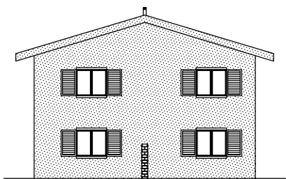
Prospetto Nord
